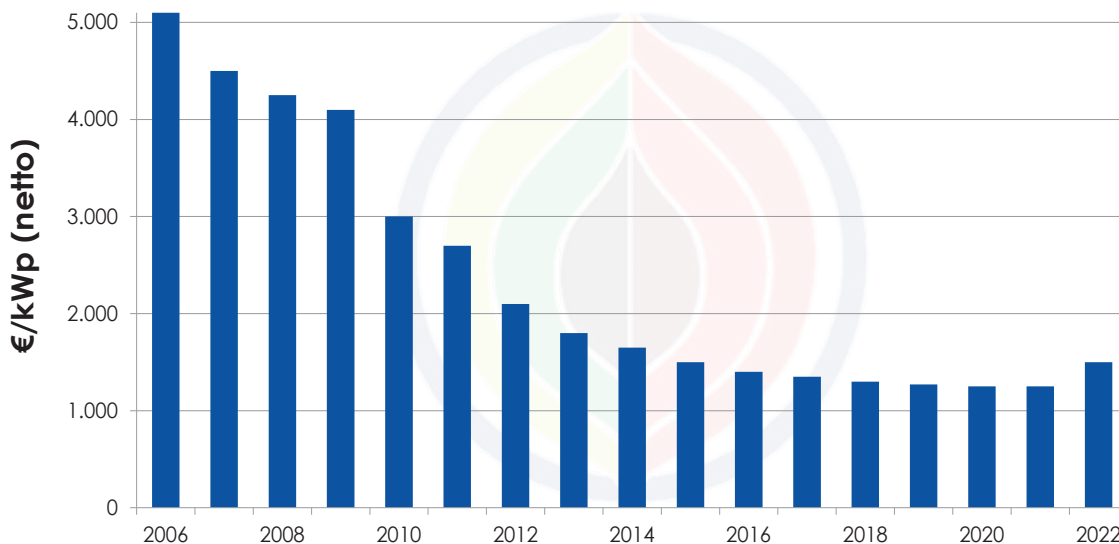
Abb. 4: Netto-Installationskosten für schlüsselfertige PV-Anlagen unter 10 kWp von 2006 bis 2022 (vorläufig) (eigene Abbildung nach eigenen Daten sowie Bundesverband Solarwirtschaft e.V. 2016; Fraunhofer ISE 2020; scon-marketing GmbH 2020 & ub.de Fachwissen GmbH o.J.)
