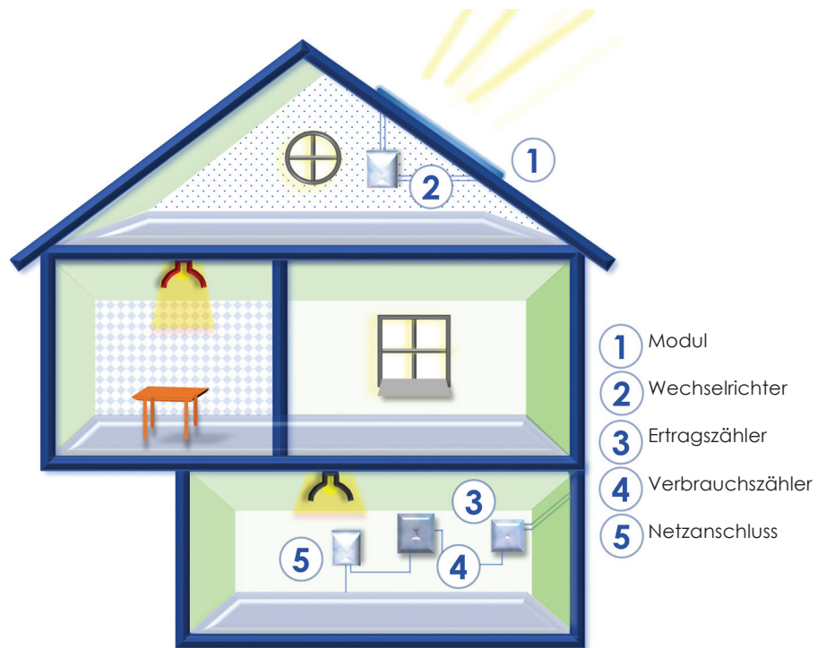
Abb. 1: Konventionelle, netzgekoppelte PV-Dachanlage
